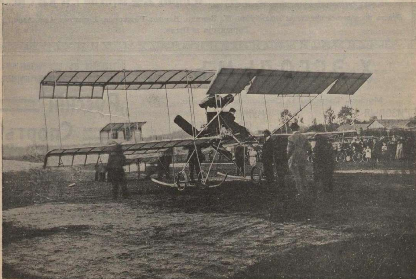
С. И. Уточкинъ на первомъ русскомъ бипланѣ, построенномъ на заводѣ „Духъ“ Ю. А. Меллера въ Москвѣ.
